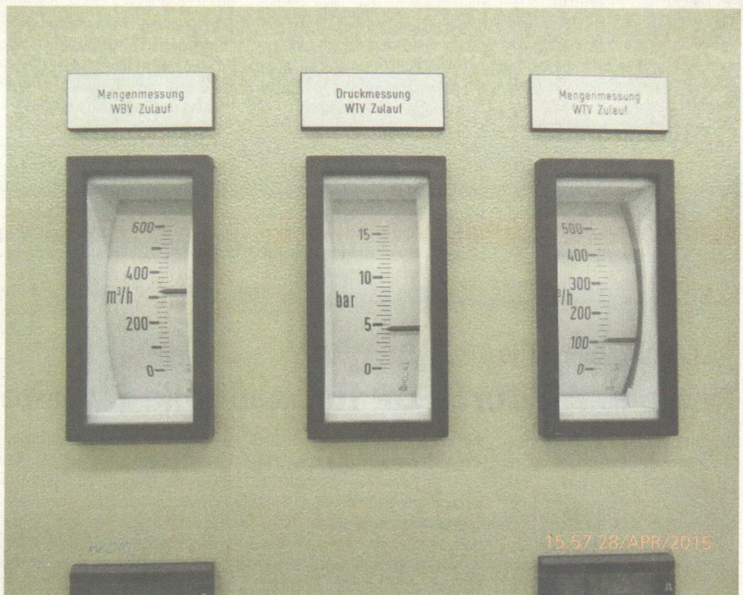
Anzeige Mischungsverhältnis im Wasserwerk
